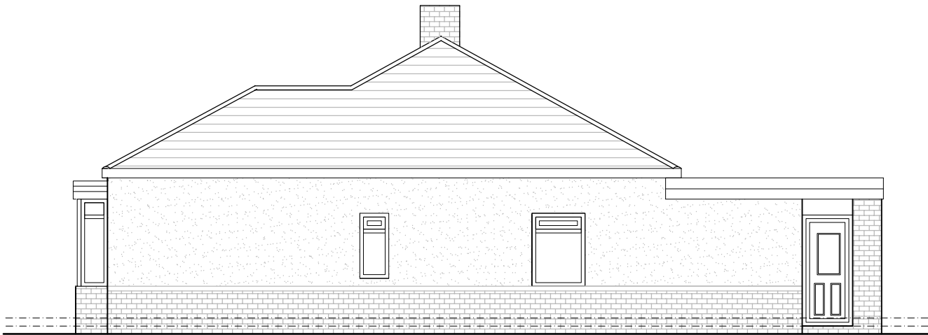
E101 Existing Right Elevation 1:100
